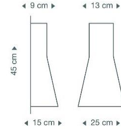
ARTEMİS-APLİK-SMALL
